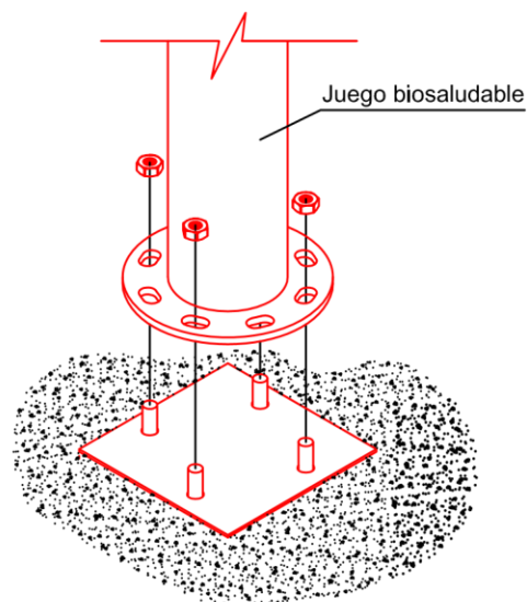
Detalle Instalación
