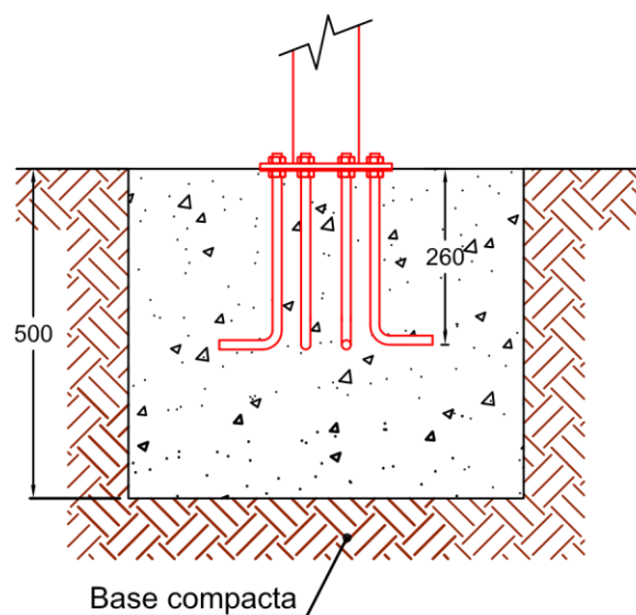
DETALLE ZAPATA
