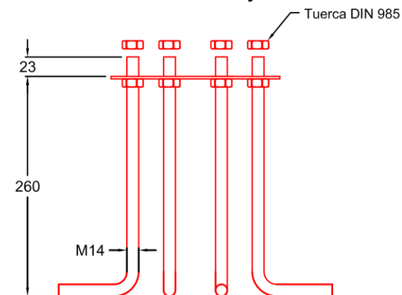
Detalle Anclaje
