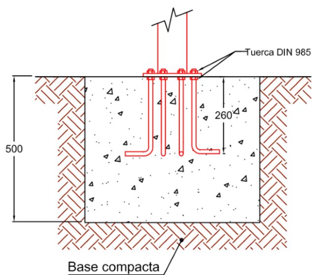
DETALLE ZAPATA
