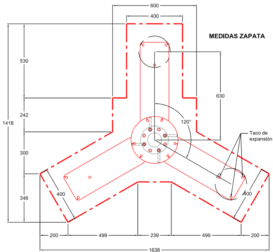
DETALLE ZAPATA
