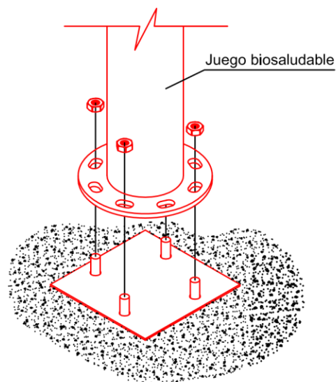
Detalle Instalación
