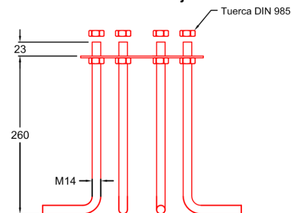
Detalle Anclaje
