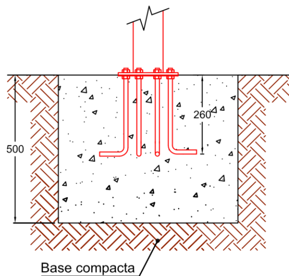
DETALLE ZAPATA
