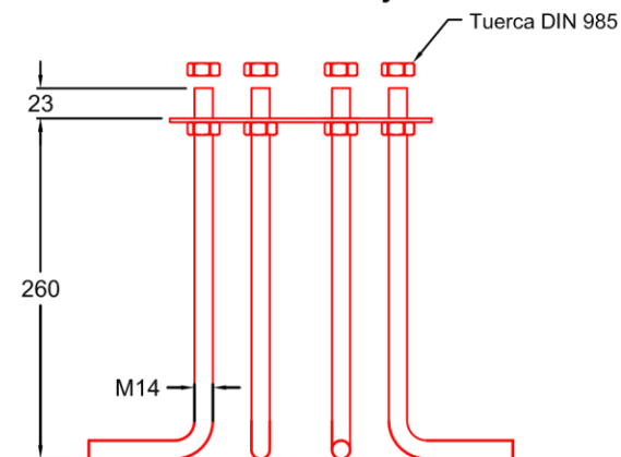
Detalle Anclaje
