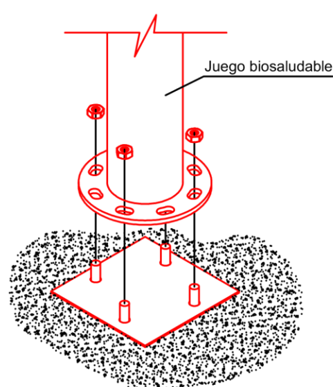
Detalle Instalación
