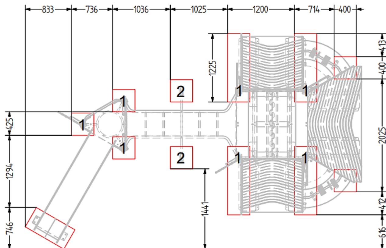
LINEA SAFARI TIPOLOGIA DE BASES PARA ARENERO
