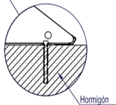
DETALLE DE CIMENTACIÓN
